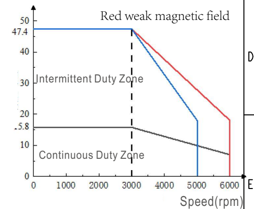
Torque(Nm)
