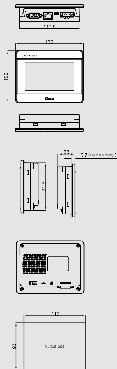
Dimension(Unit:mm)
